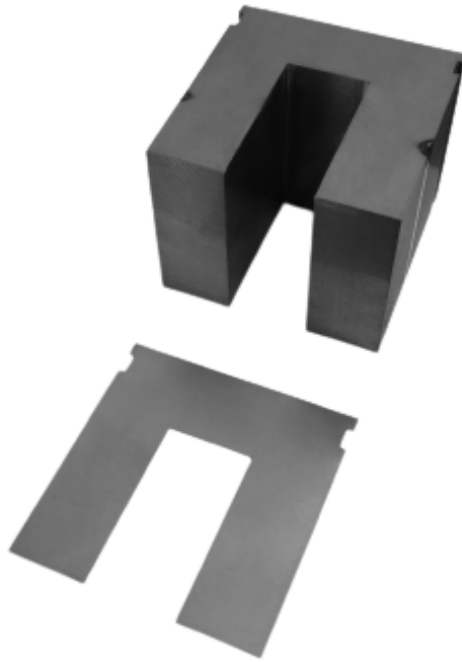
Lâminas U/ C e Núcleo soldado
